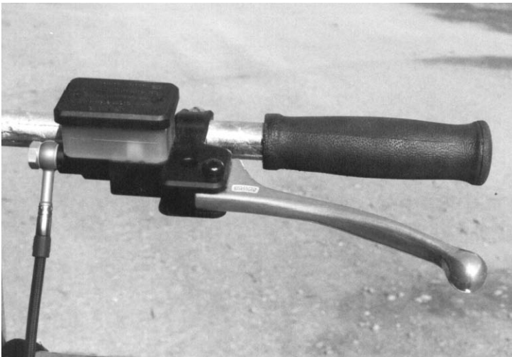
Photo N° 9 Poignée de frein hydraulique.
